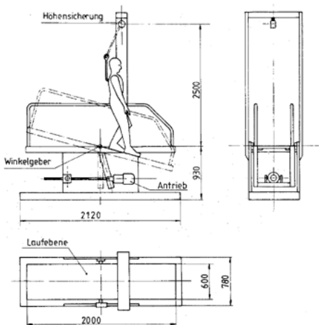
Bild 2: Prüfeinrichtung (schiefe Ebene)
