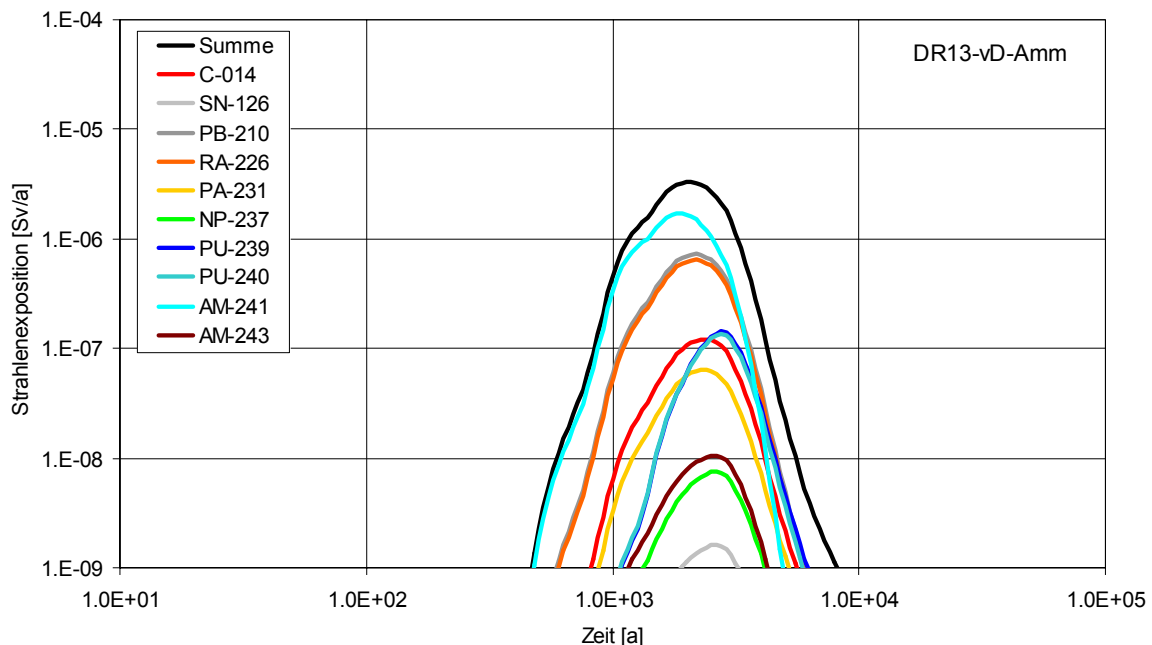
Abb. 3.67 Radionuklidbeiträge zur potenziellen Strahlenexposition für das Exfiltrationsgebiet ‚verstürztes Deckgebirge – Ammerbeek‘
