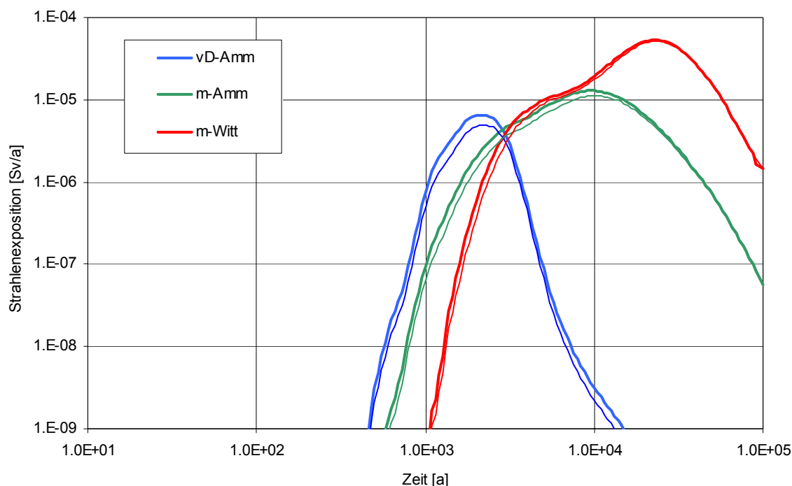
Abb. 5.102 Potenzielle Strahlenexposition für die Exfiltrationsgebiete (RX.13 vs. kombinierte Variante RX.5, dünn)
