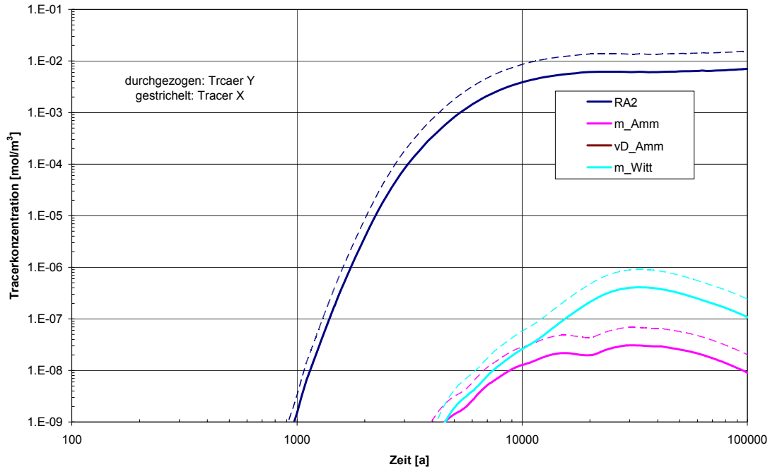
Abb. 3.32 Konzentrationen der Tracer aus LAW4 nach dem Übertritt in das Deckgebirge (RA2) und in den drei Exfiltrationsgebieten (Rechenfall RX.1-K, Tracerkonzentration in vD-Amm <1 \cdot 10^{-9} mol/m 3 )
