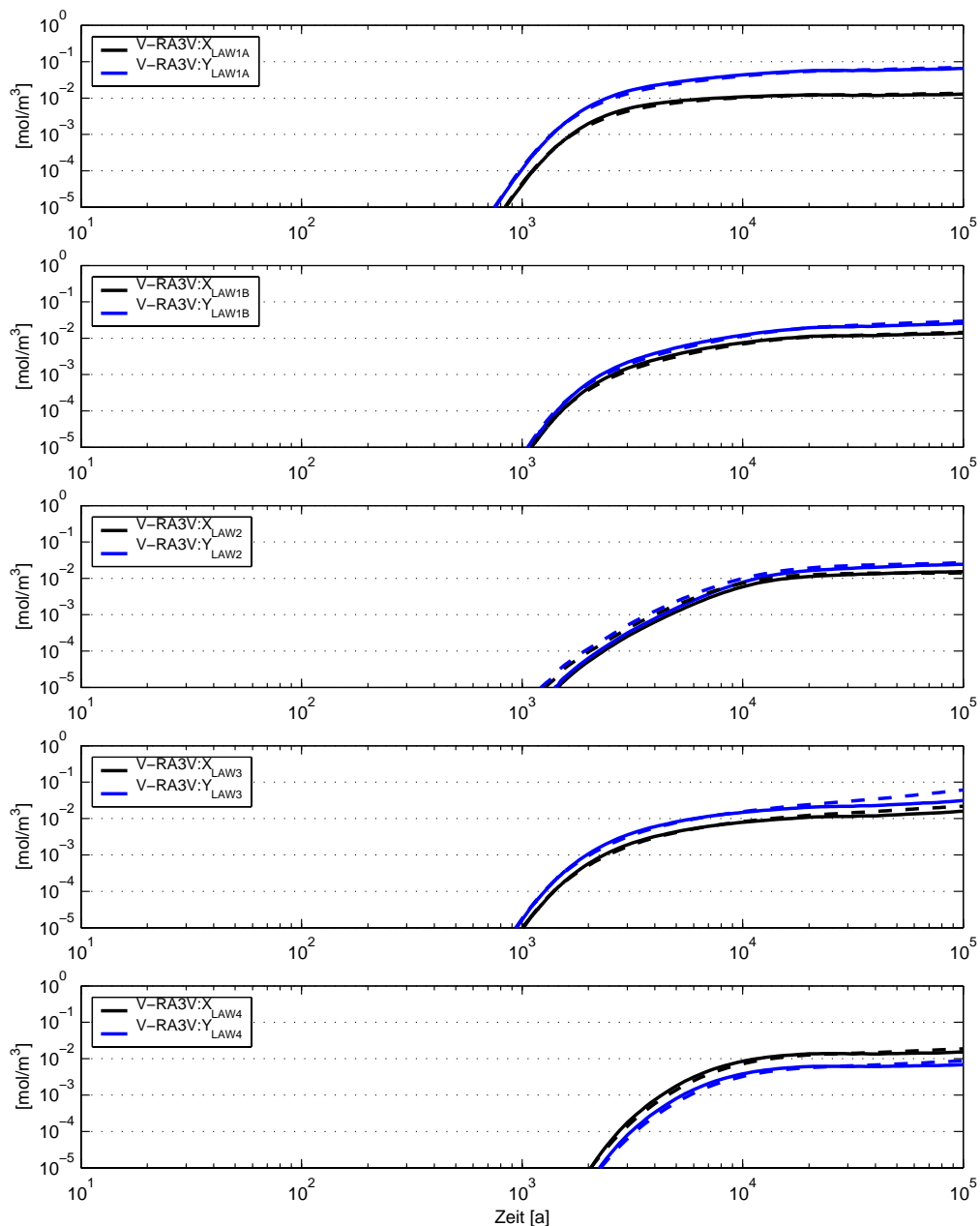
Abb. 3.27 Konzentration der Tracer X_{ELB} und Y_{ELB} im Rötanhydrit (Vergleichsfall vs. Referenzfall R8-K – gestrichelt)
