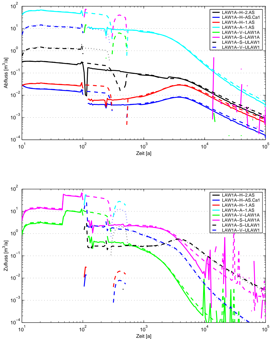
Abb. 5.28 Lösungsabfluss aus (obern) und Zufluss zu (unten) LAW1A in RX.5-K
