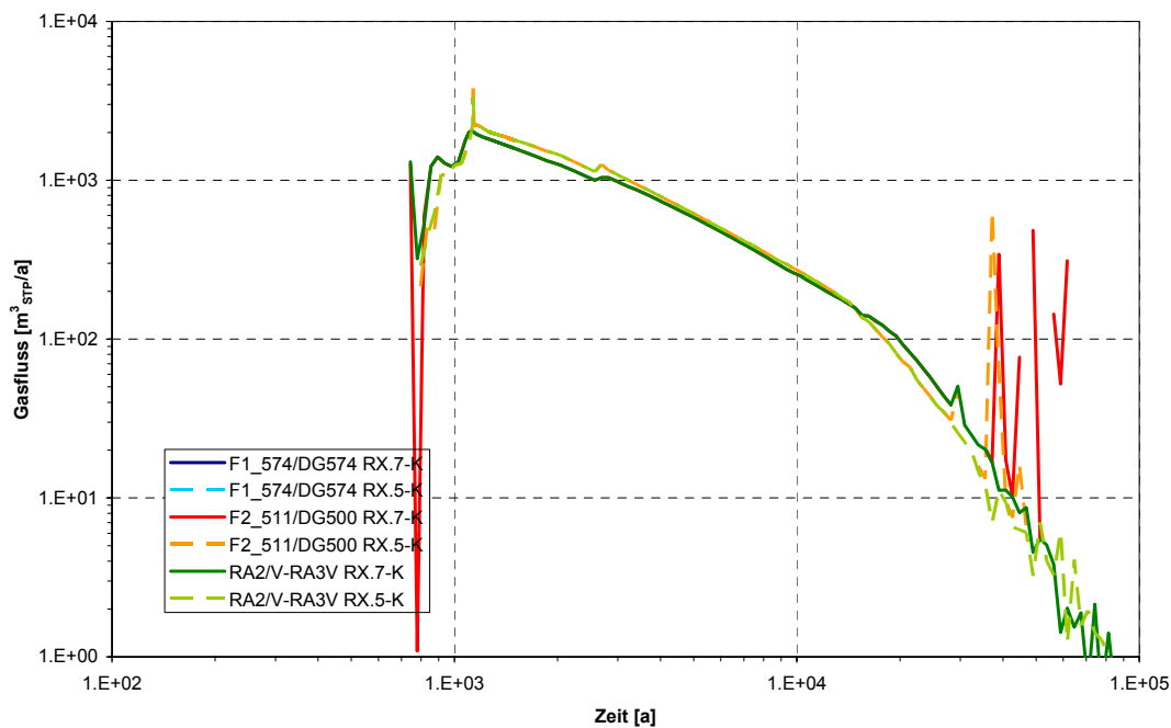
Abb. 5.74 Gasabfluss ins Deckgebirge in RX.7-K, z. Vgl. gestrichelt RX.5-K (oben linear, unten logarithmisch)
