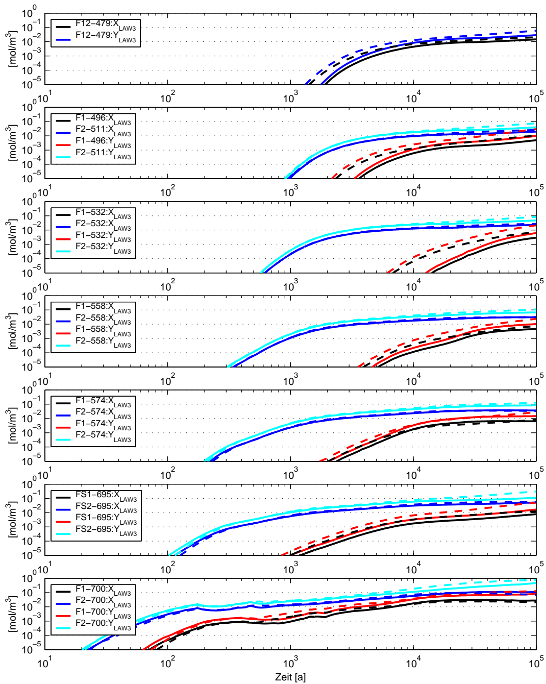
Abb. 3.23 Tracerkonzentrationen X_{LAW3} und Y_{LAW3} in der Südflanke (Vergleichsfall vs. Referenzfall R8-K – gestrichelt)
