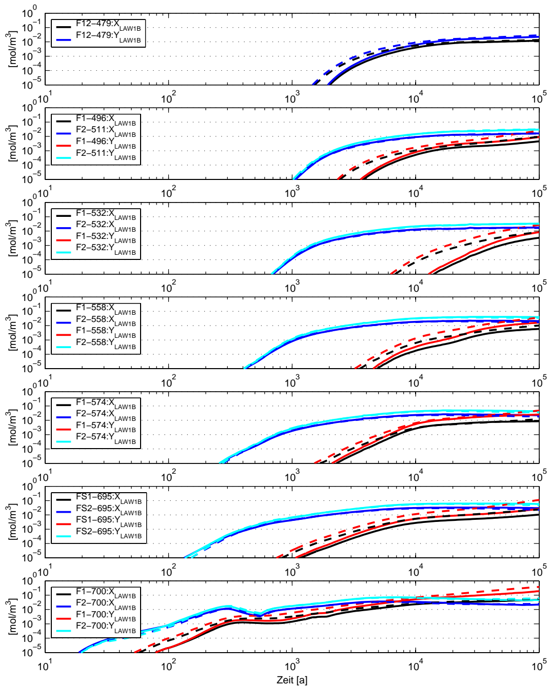
Abb. 3.21 Tracerkonzentrationen X_{\text{LAW1B}} und Y_{\text{LAW1B}} in der Südflanke (Vergleichsfall vs. Referenzfall R8-K – gestrichelt)
