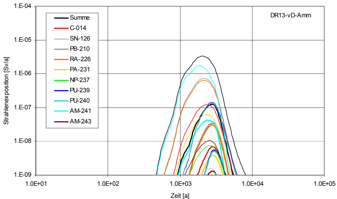
Abb. 4.15 Nuklidbeiträge zur potenziellen Strahlenexposition für das Exfiltrationsgebiet ‚verstärktes Deckgebirge – Ammerbeek‘ (SFKan80% vs. Vergleichsfall RX.1, dünn)
