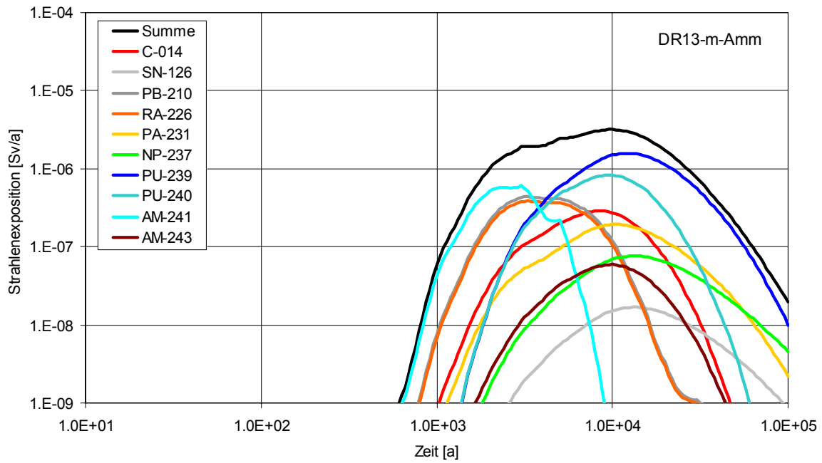
Abb. 3.68 Radionuklidbeiträge zur potenziellen Strahlenexposition für das Exfiltrationsgebiet ‚Muschelkalk – Ammerbeek‘
