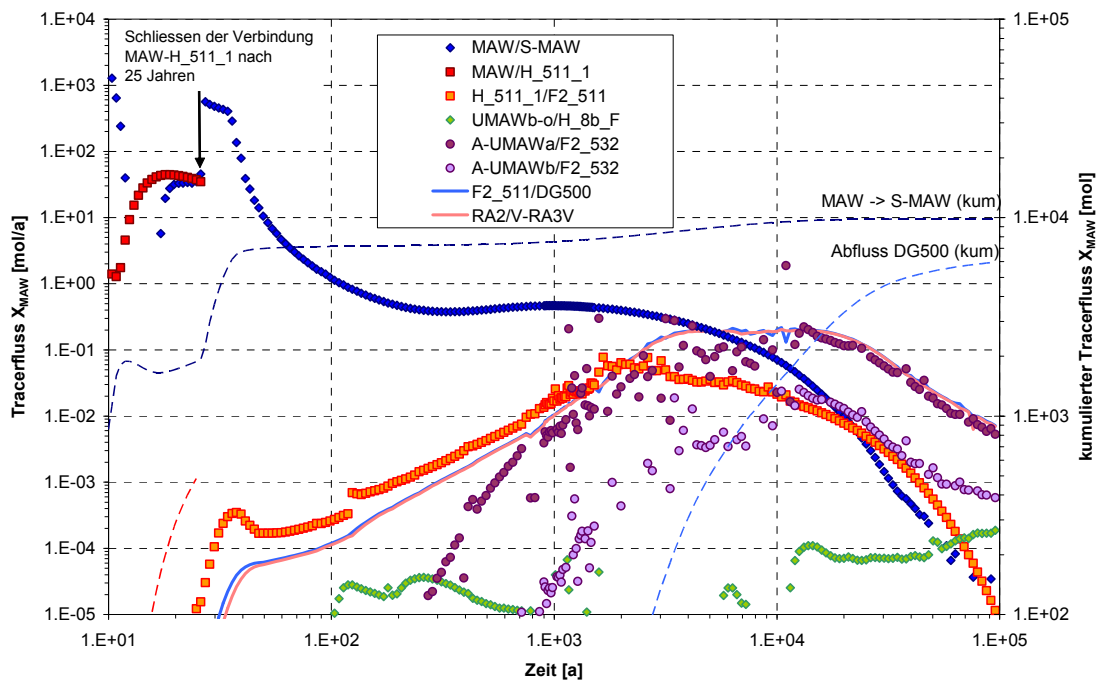
Abb. 5.149 Fluss des Tracers X_{MAW} im Nahbereich der MAW, im Baufeld in der Südflanke und im Deckgebirge; gestrichelt kumulierter Tracerfluss: Variante RIX.2-K
