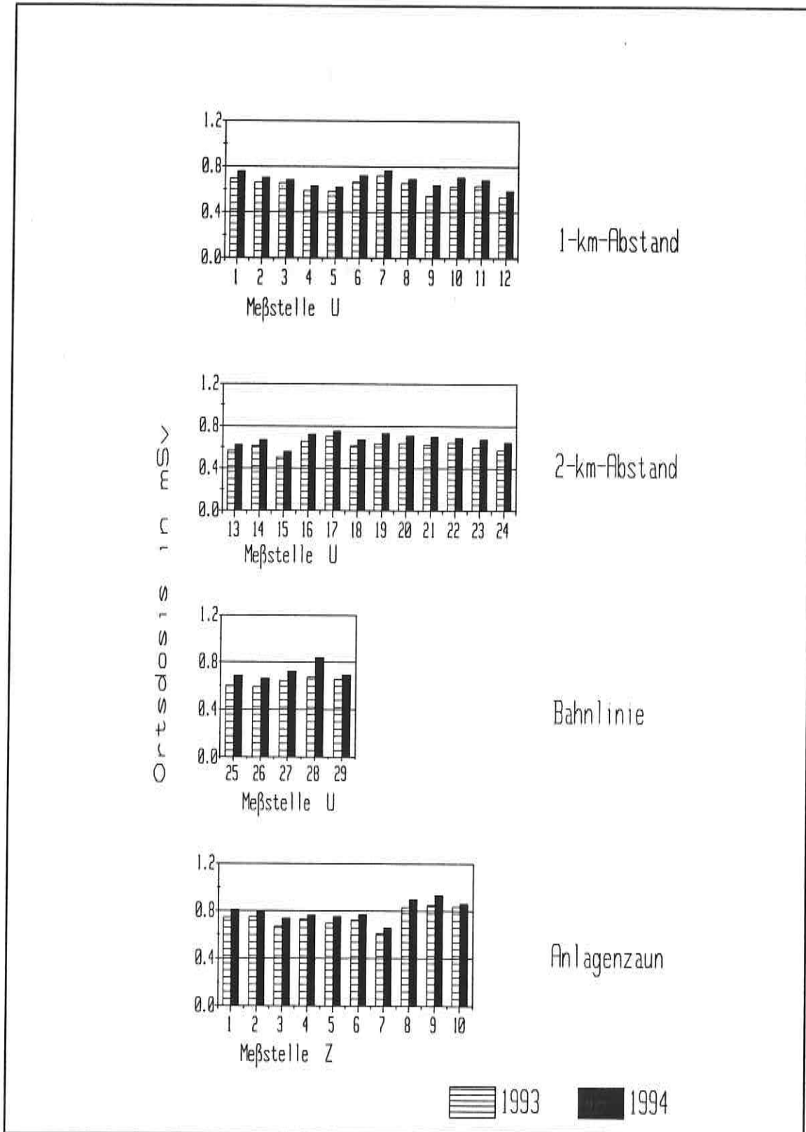
Abb. 5: Jahres-Ortsdosis gem. Tabelle 7 in der Umgebung der Schachtanlage Asse 1993 und 1994. Lage der Meßstellen Z und U lt. Abb. 3 und Abb. 4
