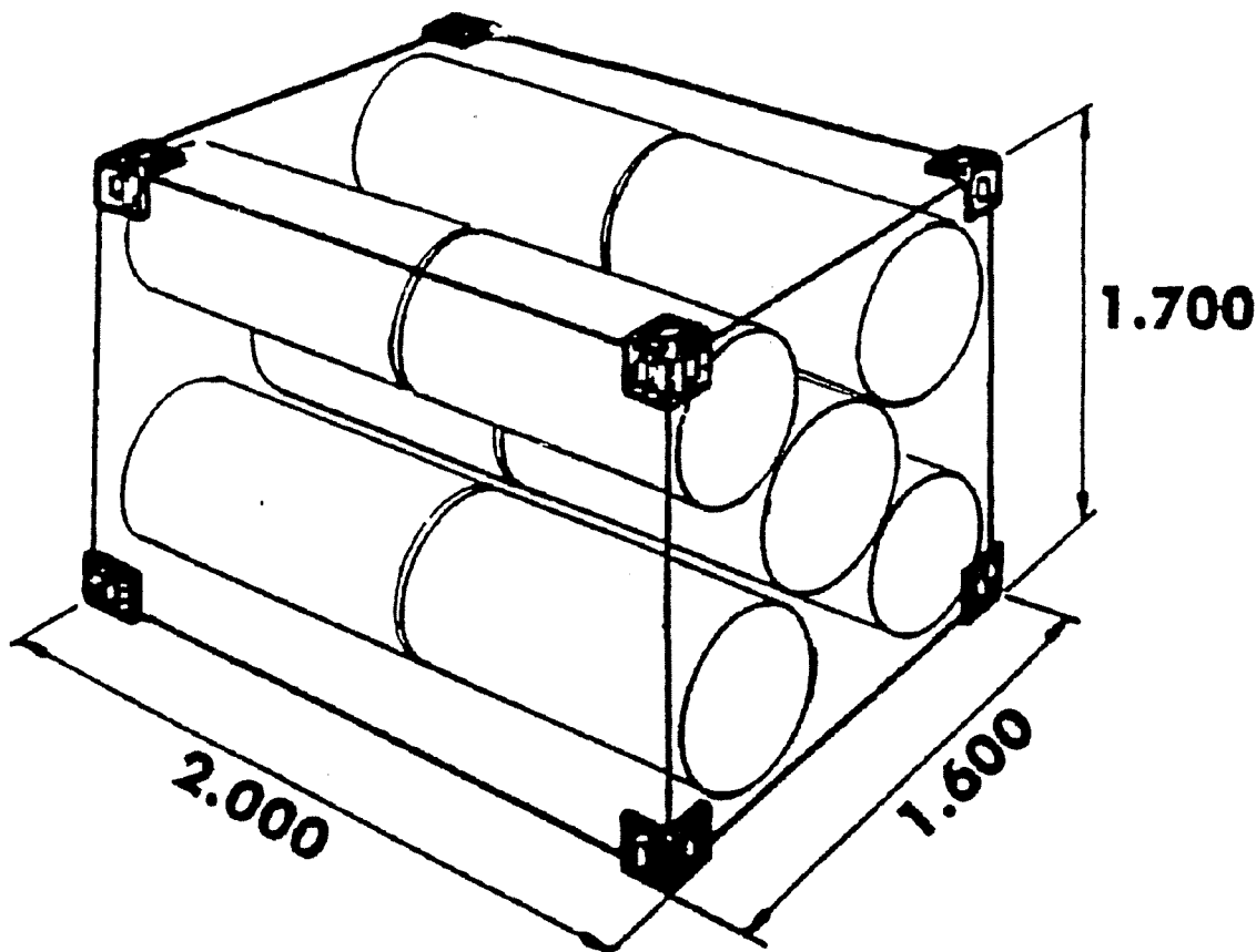
Abb. 5: Befüllung des Containers Typ VI mit 10 Fässern (nach /12/)
