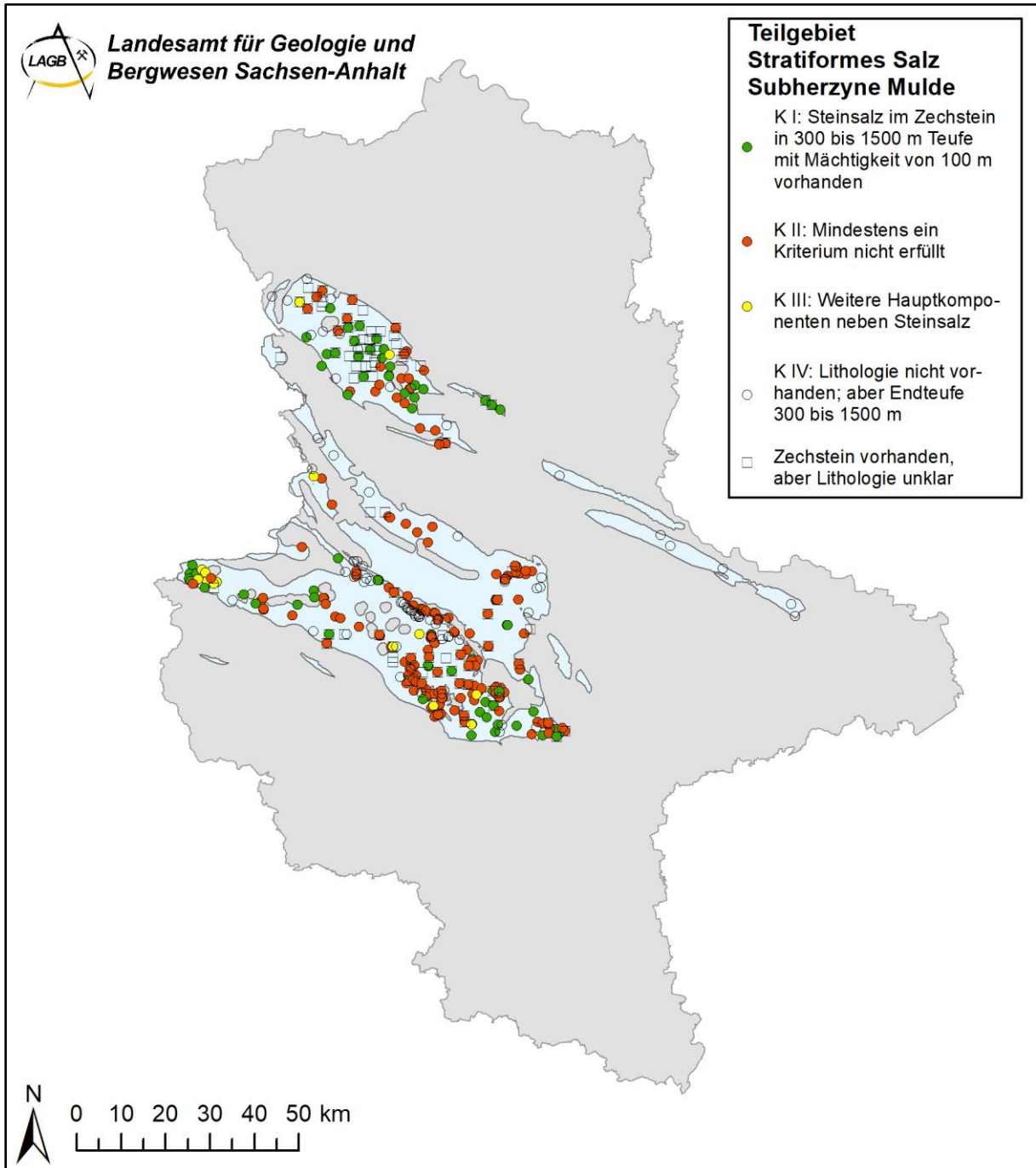
Abb. 7: Teilgebiet 078_05TG_197_05_IG_S_f_z. Stratiform-gelagertes Salz in der Subherzynen Mulde in Sachsen-Anhalt dargestellt mit dem lithologischen Ansatz für das Wirtsgestein Steinsalz.
