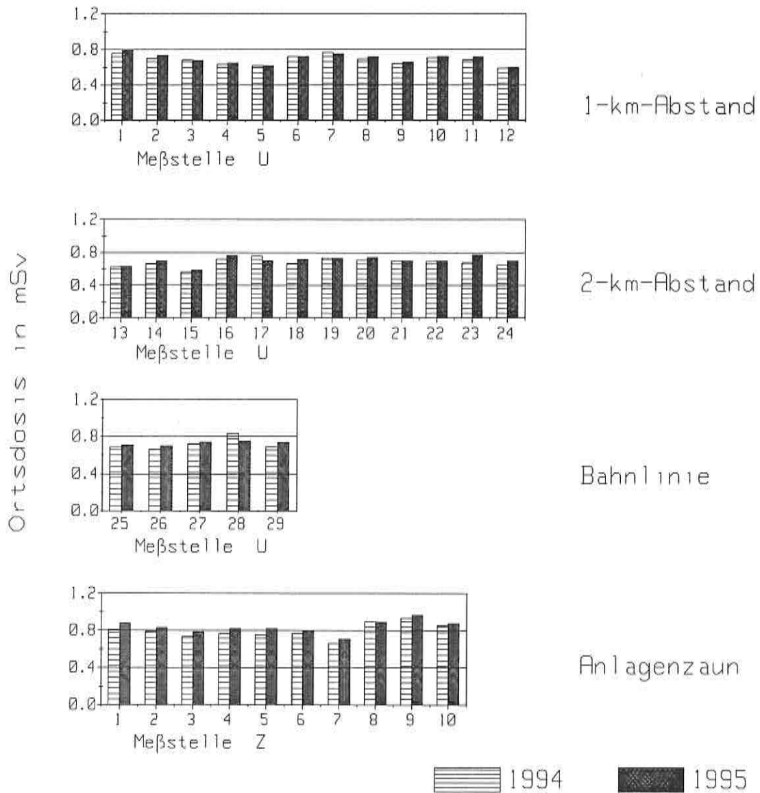
Abb. 5: Jahres-Ortsdosis gem. Tabelle 7 in der Umgebung der Schachtanlage Asse 1994 und 1995. Lage der Meßstellen Z und U lt. Abb. 3 und Abb. 4
