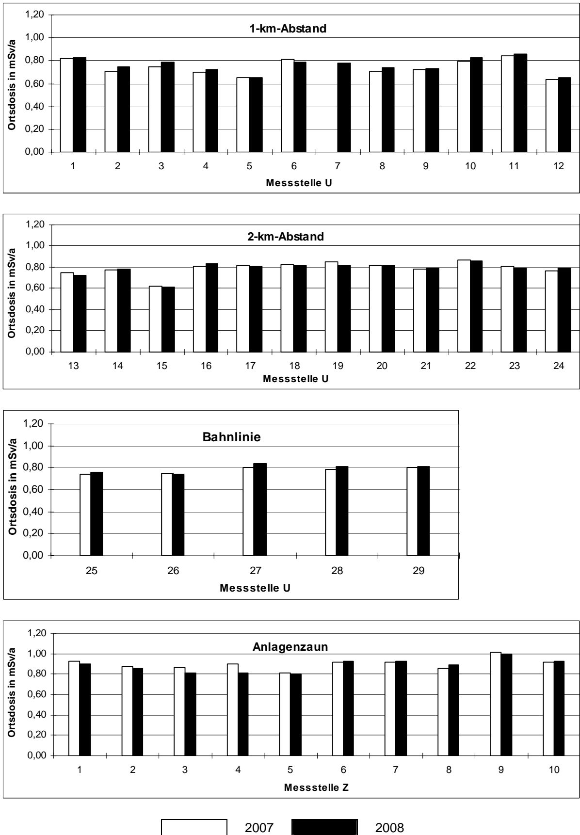
Abbildung 5: Jahresortsdosis gem. Tabelle 7 für die Jahre 2007 und 2008 in der Umgebung der SchachanlageASSE, Lage der Messstellen Z und U vgl. Abbildung 3 und Abbildung 4
