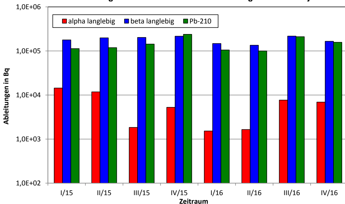
Abb. 3.1.4: Aerosolableitungen mit den Abwettern 2016 im Vergleich zum Vorjahr
