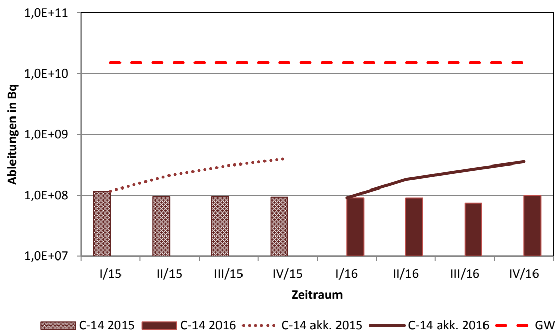
Abb. 3.2.2: C-14 (als ^{14}\text{CO}_2 ) - Ableitungen mit den Abwettern 2016 im Vergleich zum Vorjahr
