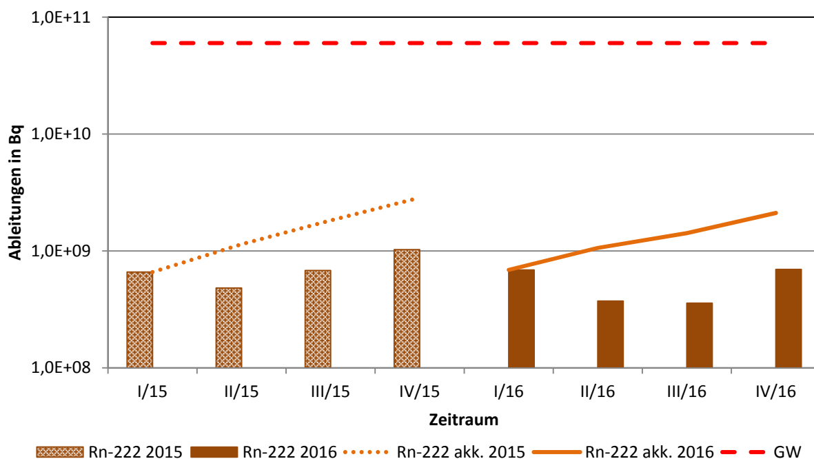
Abb. 3.1.3: Rn-222 (EEC) (kurzlebige Aerosole) - Ableitungen mit den Abwettern 2016 im Vergleich zum Vorjahr
