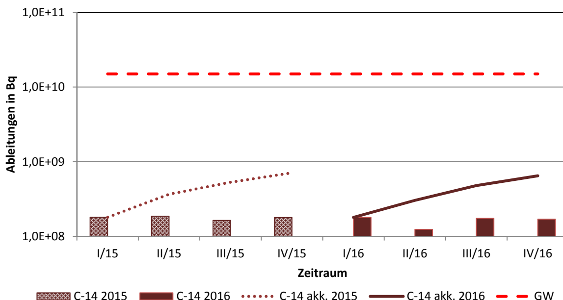
Abb. 3.1.2: C-14 (als ^{14}\text{CO}_2 ) - Ableitungen mit den Abwettern 2016 im Vergleich zum Vorjahr
