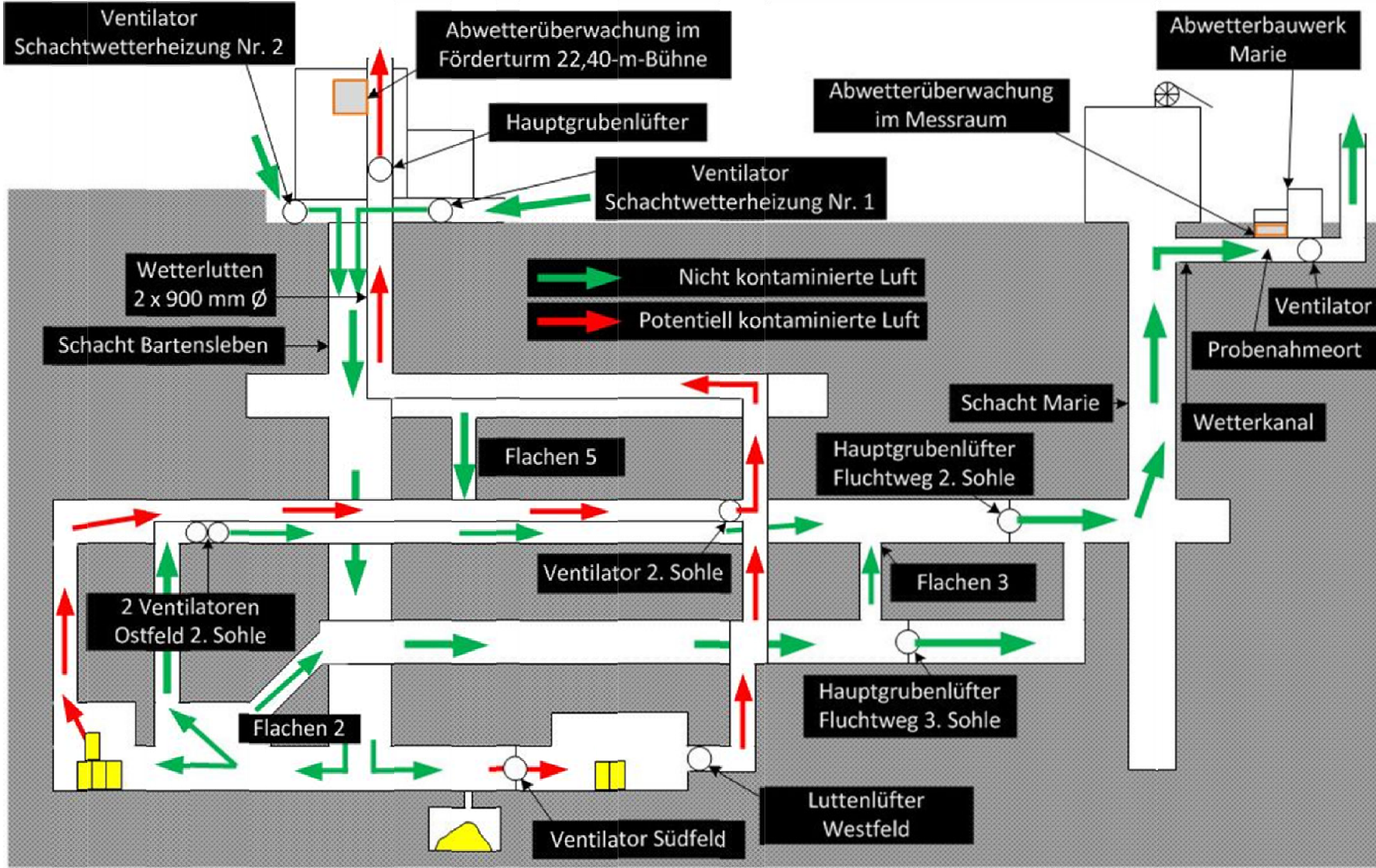
Abb. 2.1: Schematische Darstellung der Bewetterung der Einlagerungsbereiche
