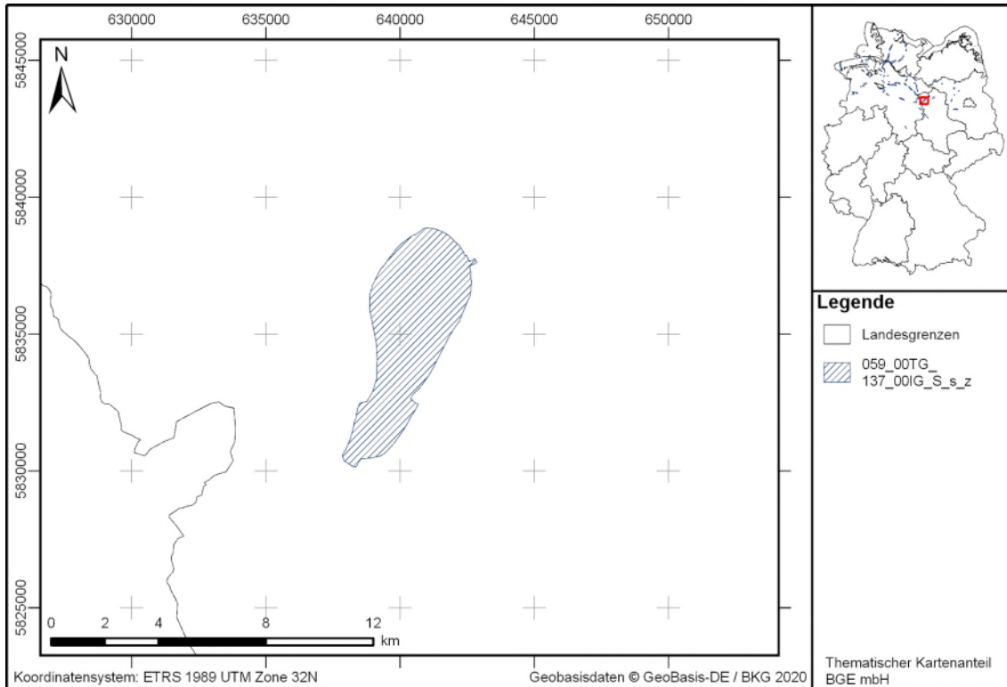
Abbildung 1: Übersichtskarte des Teilgebiets 059_00TG_137_00IG_S_s_z
